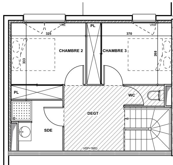
PLAN ETAGE
