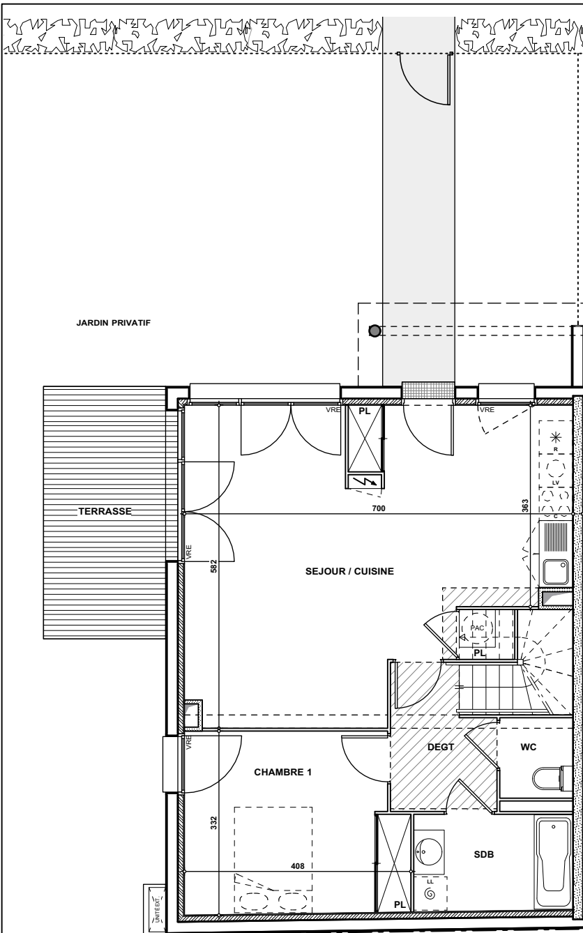
PLAN RDC
